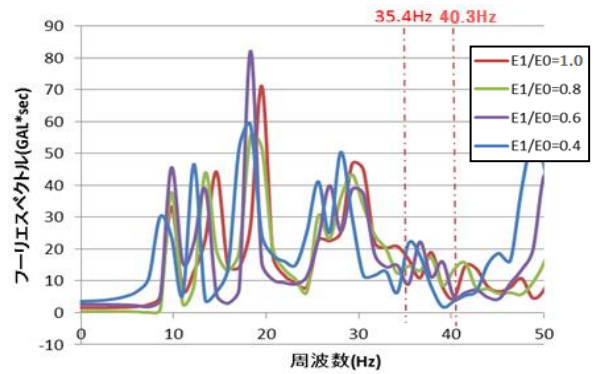
図-4 着目点 7 における振幅スペクトル
