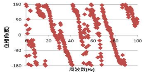
図-3 着目点7における実測位相差スペクトル
