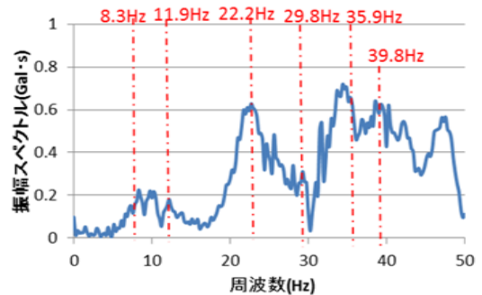
図-2 着目点7における実測振幅スペクトル
