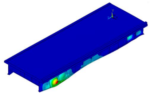
(1) 全体モード図
