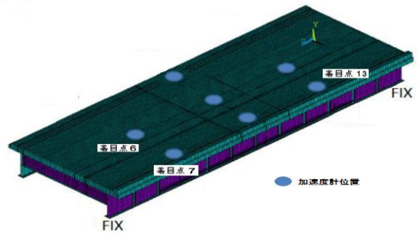
図-1 対象橋梁のFEM解析モデルと着目点
