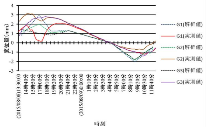
図 - 7 鉛直変位の実測値と解析値
