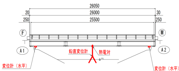
図-1 側面図・計測器設置概要図
