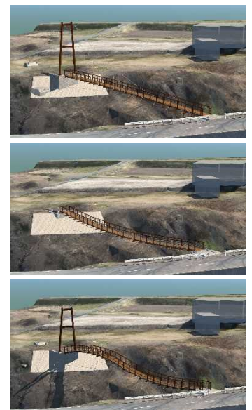
図-4 吊橋構造デザイン
