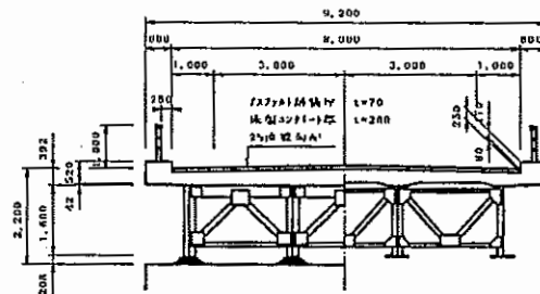
図-2. 有根橋の断面
