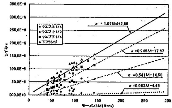
図-4. 有根橋の曲げモーメントとひずみの関係
