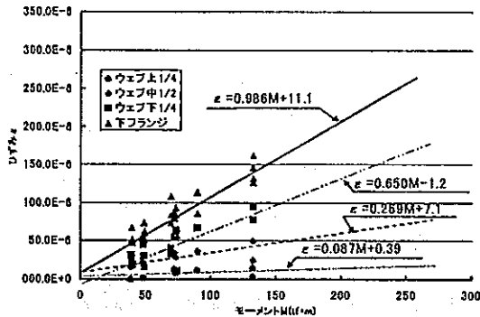
図-3. 正徳橋の曲げモーメントとひずみの関係
