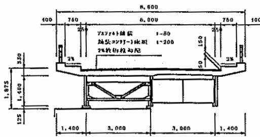
図-1. 正徳橋の断面
